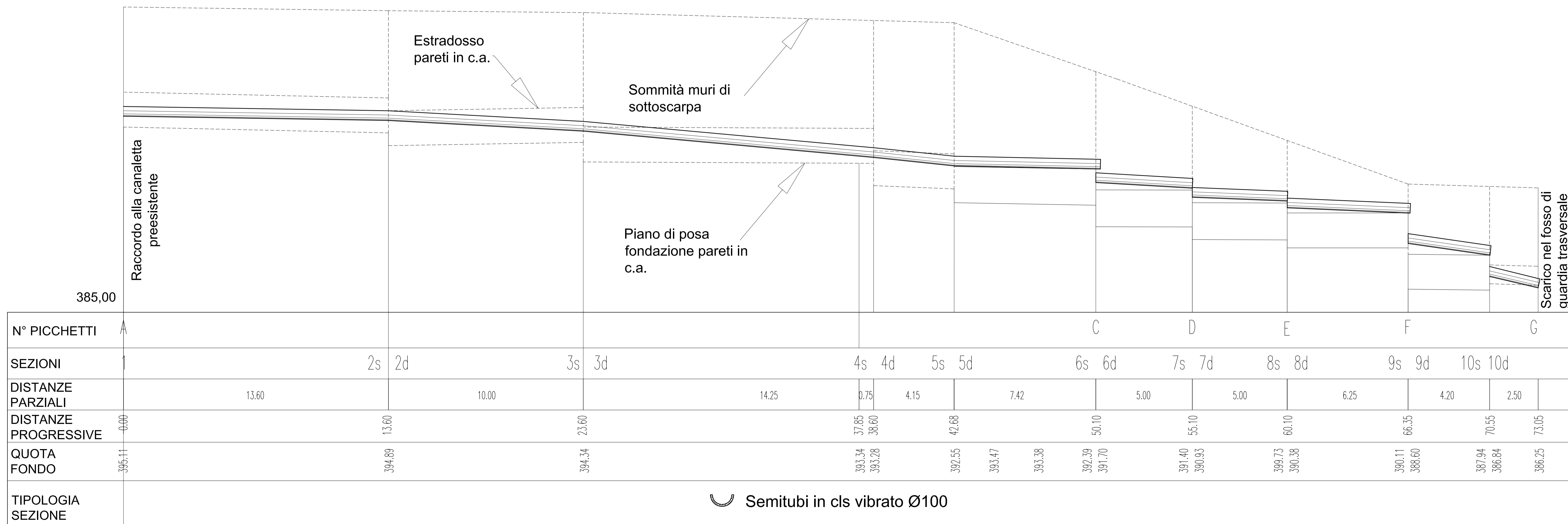
PROFILO LONGITUDINALE NUOVA CANALETTA REALIZZATA
